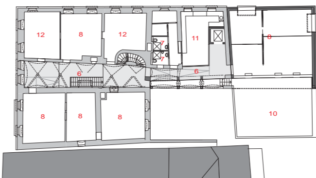
一樓平面圖 FRIST FLOOR PLAN
